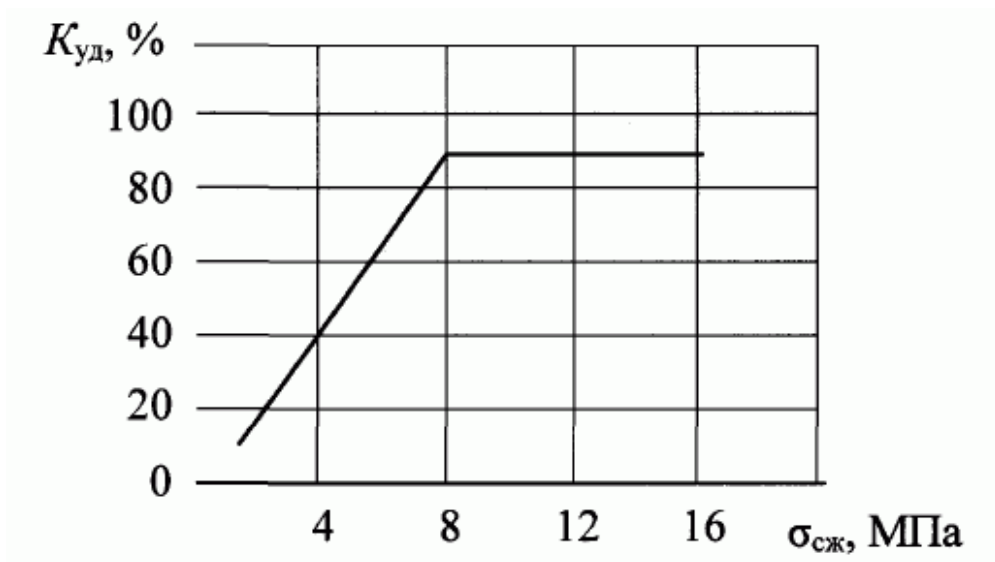
Рис. 1. График зависимости K_{уд} от \sigma_{сж} .
