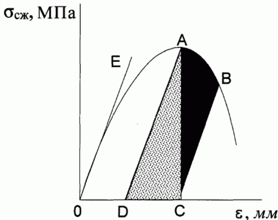
Рис. 2. График зависимости \sigma_{сж} от \epsilon .
